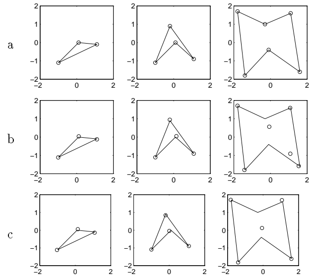
Fig. 1 : Les résultats de reconstructions avec différents paramètres : - Objet initial, o Les sommets reconstruits.
