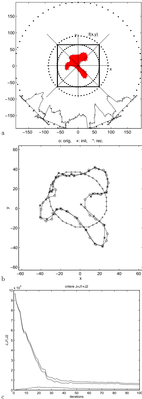
Fig. 2: Reconstruction tomographique pour une application en CND.
